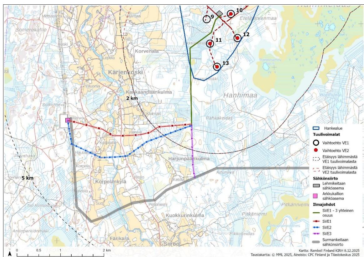
Kuva 4-2. Hankkeen sähkönsiirtoreittivaihtoehdot.
